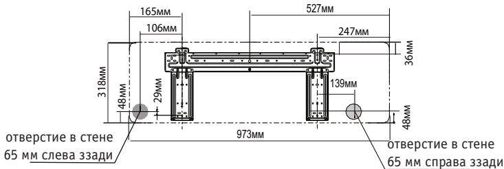
Типоразмер D
